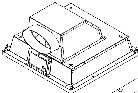
Fan Module
